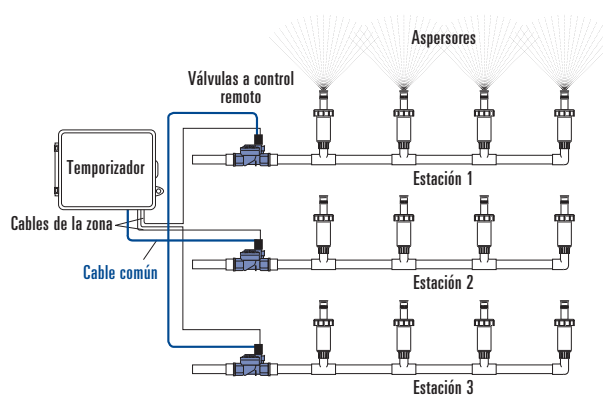
Figura 13: Conexión de los cables del aspersor a las válvulas
